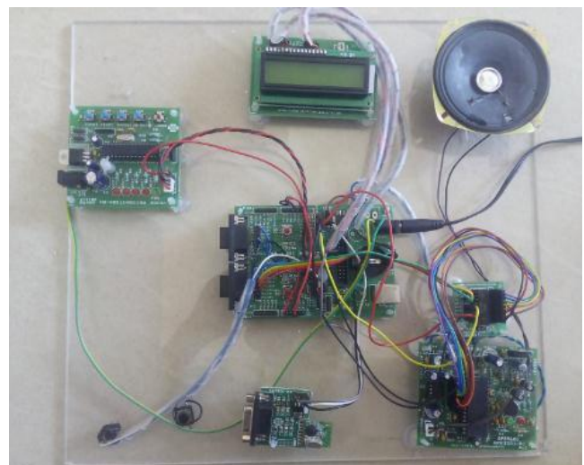
Fig 4: Blind module.
