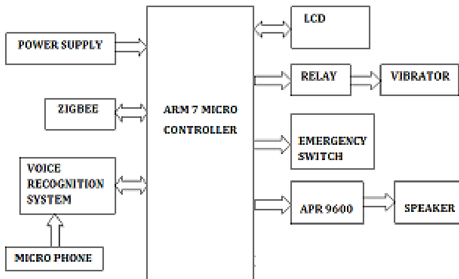
Fig 1: Blind unit.
